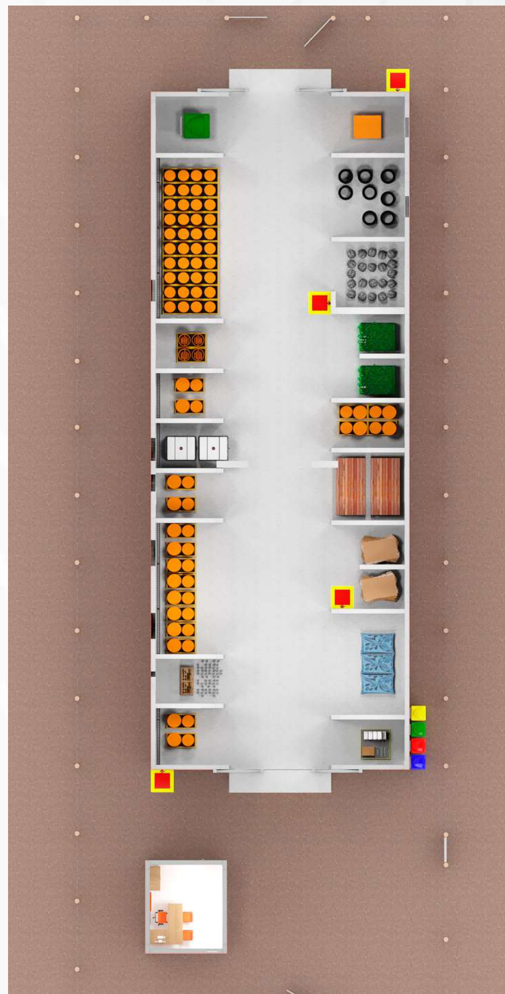
Projeto de galpão de estocagem de resíduos perigosos e não perigosos para área industrial de siderurgia.
